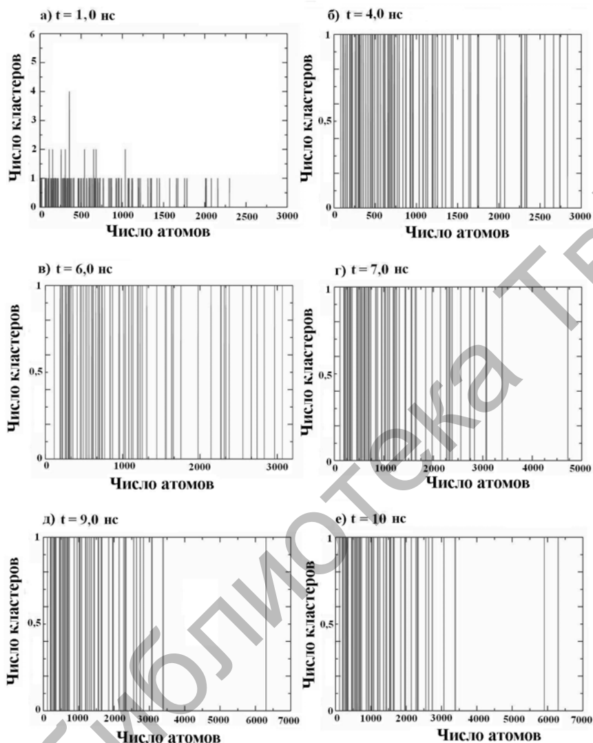
Рис. 2. Распределение кластеров по размеру для системы из 85000 атомов N_i в зависимости от времени процесса синтеза.
