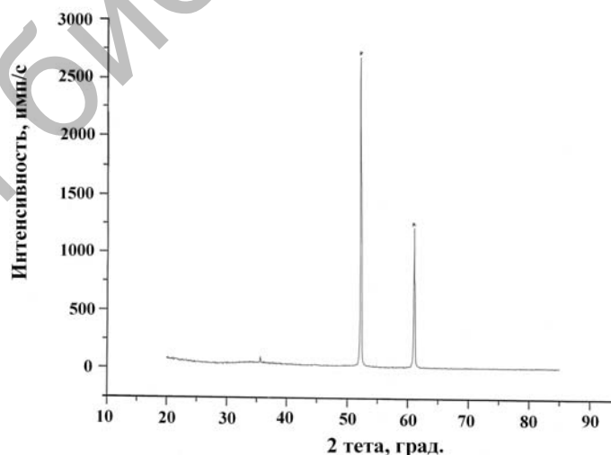
Рис. 1. Данные рентгенографического исследования полученного нанопорошка никеля (при \text{Co} -излучении)
