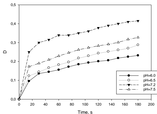
Зависимость оптической плотности от времени с разными рН
