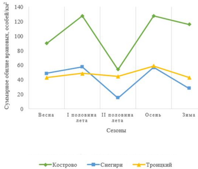
Рис. 2. Среднезональное обилие врановых в посёлках северо-западного Подмосковья
