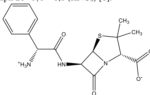
Цвиттер-ион ампициллина
