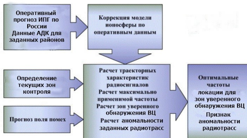
Рис. 8: Структурная схема проведения точного прогноза характеристик радиотрасс на основе гелиогеофизических данных
