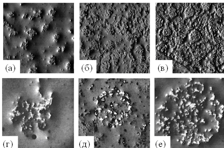
Р и с . 1 . АСМ-изображения СУА-вулканизатов СКЭПТ-4044, [S] = 0.5 (а), 1.0 (б), 1.5 мас.ч. (в). Размер изображений 30х30 (а-в) и 5х5 мкм (г-е)
