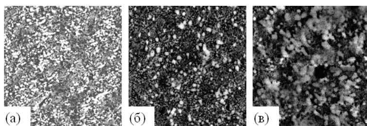
Р и с . 2 . АСМ-изображения СУА-вулканизатов СКЭПТ-4535, [S] = 0.5 (а), 1.0 (б), 1.5 мас.ч. (в). Размер изображений 10х10 мкм.
