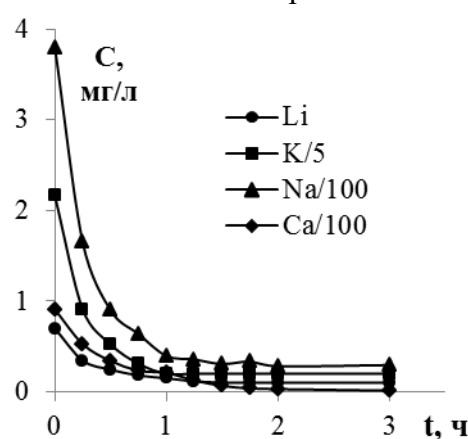
Р и с . 1 . Сорбция катионов смолой ТОКЕМ–160 из раствора Верхне-Паратунского геотермального месторождения
