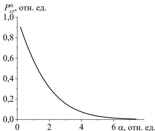
Рис. 2. Зависимость критической мощности от нормированной интенсивности излучения.
