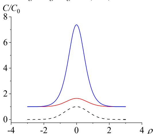
Рис. 1. Зависимость приведенной концентрации наночастиц от приведенного расстояния \rho до оси пучка для разных значений интенсивности излучения: \alpha = 0,5 (красная кривая); \alpha = 5 (синяя кривая). Для сравнения пунктиром показана координатная зависимость интенсивности излучения.
